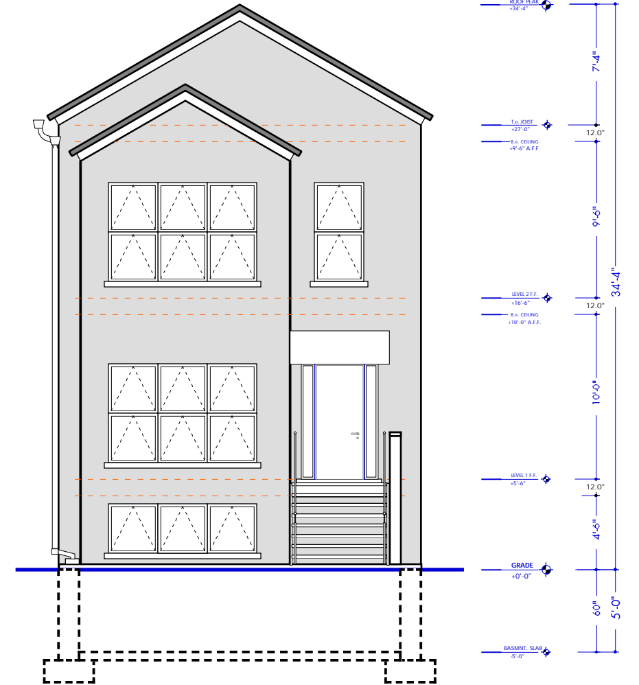
EAST ELEVATION E1
