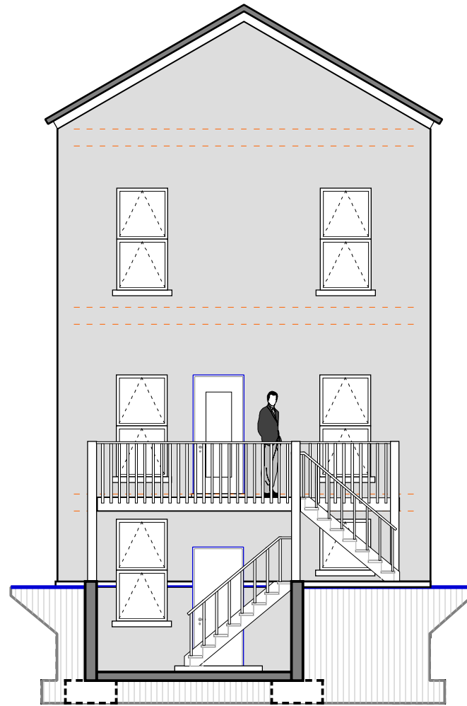
WEST ELEVATION E2
