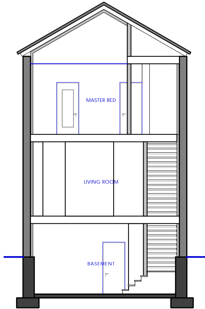
EAST SECTION E3
